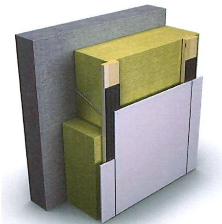
Fig. 2 Prinsipiell utførelse av PAROC ZEROfix montert på eksisterende veggkonstruksjon. Eksempel med utvendig platekledning. Figur: Paroc AB
